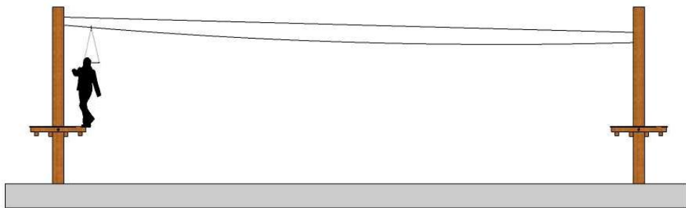
LANOVKA trenažér pro nácvik sebejištění
