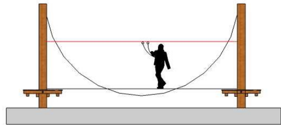
VOLNÁ UZDA trenažér pro nácvik sebejištění
